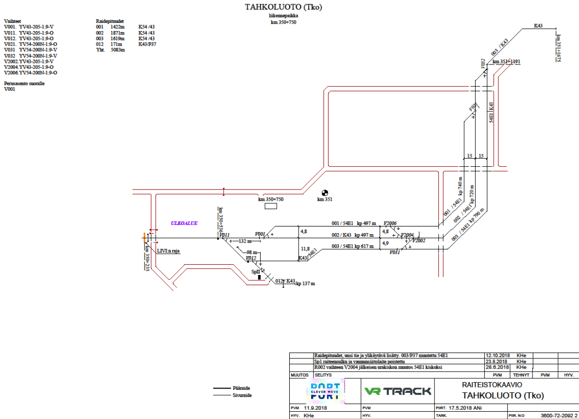
Raiteistokaavio Tahkoluoto
